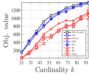
(a) Lin. reg. ( \tau = 20 )
