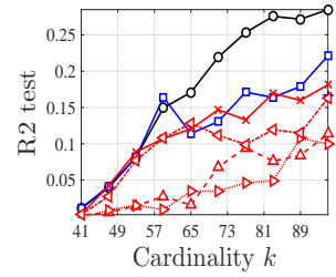
(d) Lin. reg. ( \tau = 40 )
